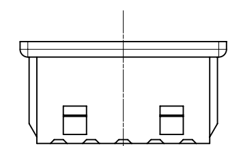
△4 2, 3極ロック形状(1ロック) FIGURE OF 2, 3 CIRCUIT (1 LOCK) △4 4極以上ロック形状(2ロック) FIGURE OF MORE THAN 4 CIRCUIT (2 LOCKS)
