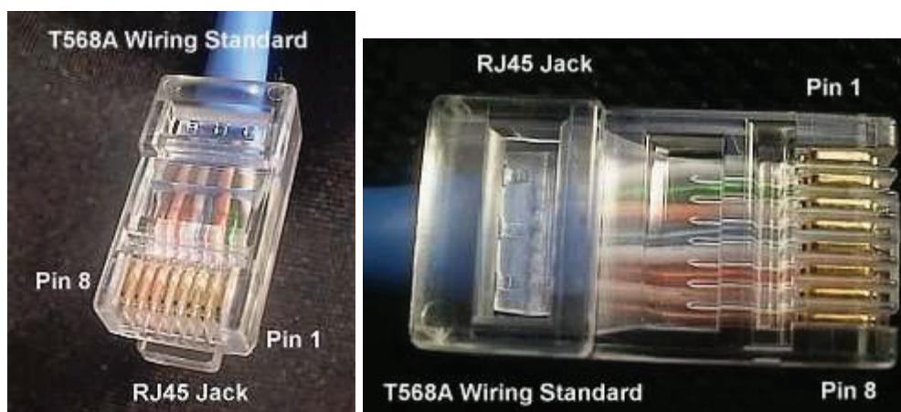
Fotografie del connettore completato.
