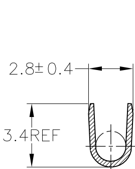
断面 A-A SECT A-A (175027のみ適用) (ONLY 175027)
